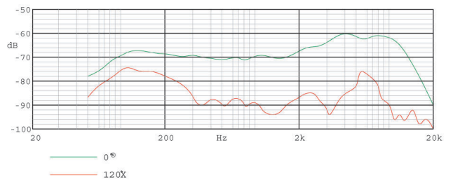
频率响应
