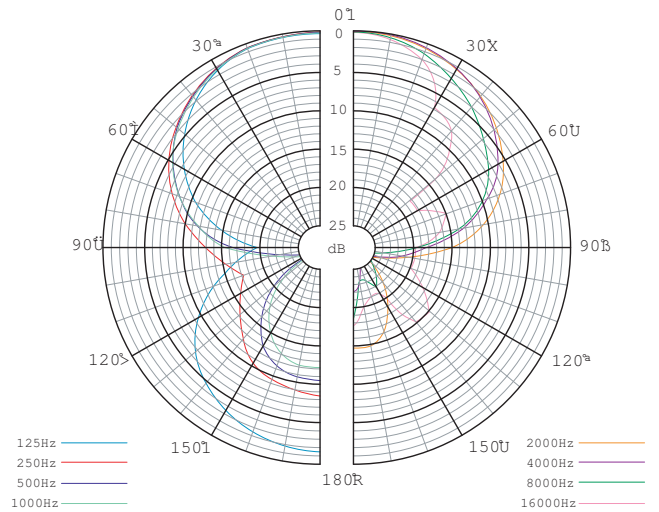
指向性图样
